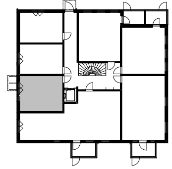
POHJAKAAVIO 1:500
