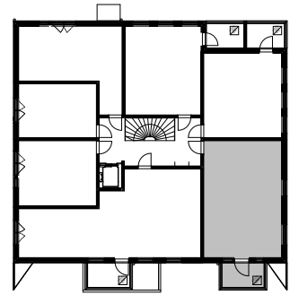
POHJAKAAVIO 1:500
