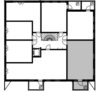
POHJAKAAVIO 1:500
