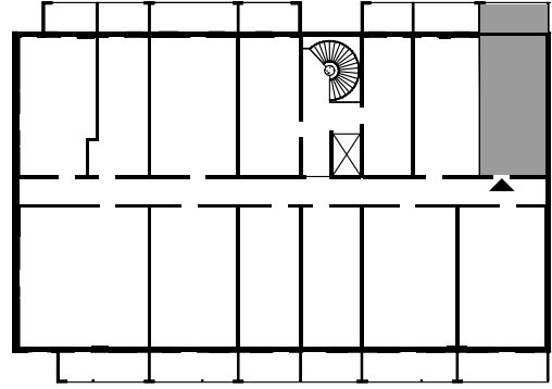
POHJAKAAVIO 1:500
