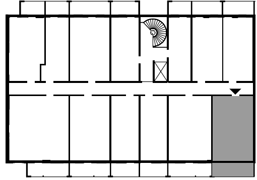
POHJAKAAVIO 1:500
